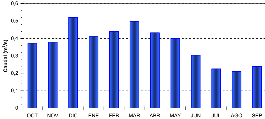
Fig. 1. Régimen anual del río Matarraña en el Aforo 052 en Beceite. (Fuente CHE)
