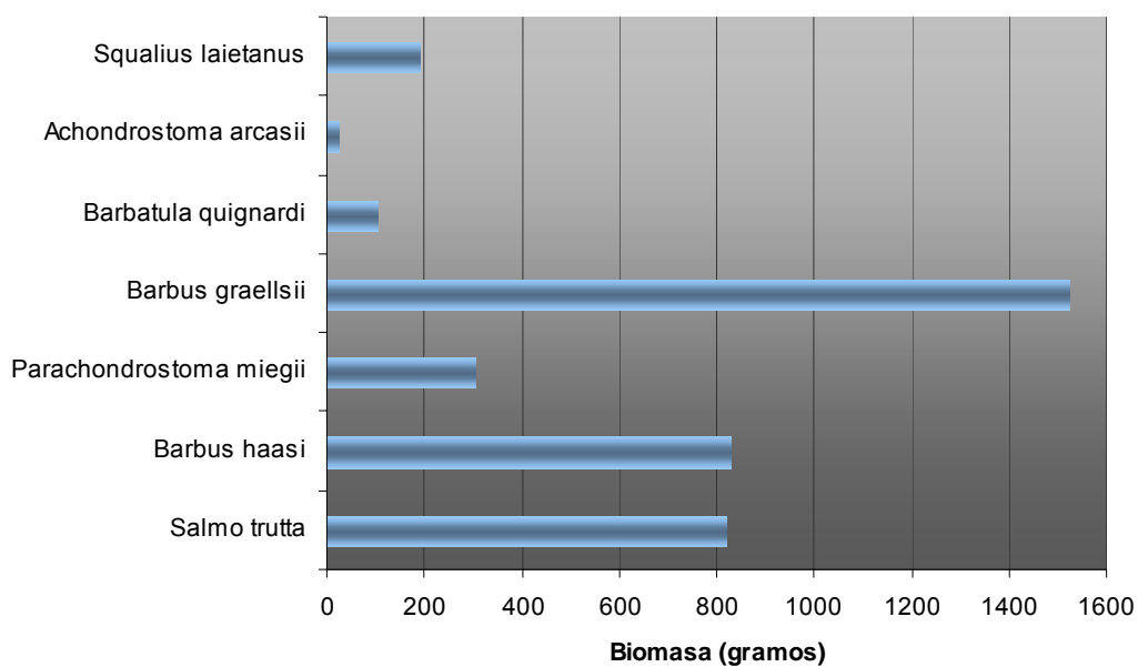
Fig. 3. Biomasa por especies en el muestreo IBI 140 del río Matarraña.
