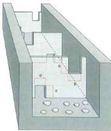
Fig. 9. Vista de una escala de estanques sucesivos. (Larínier 1992)
