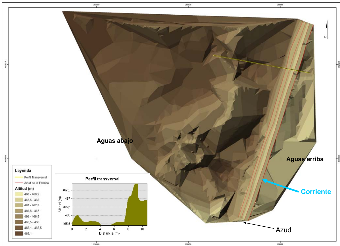
Fig. 7. Modelo Digital de Terreno y Perfil transversal del azud
