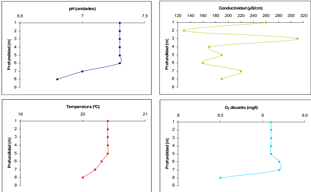
GRÁFICO 1 PERFILES FÍSICO-QUÍMICOS DEL EMBALSE
